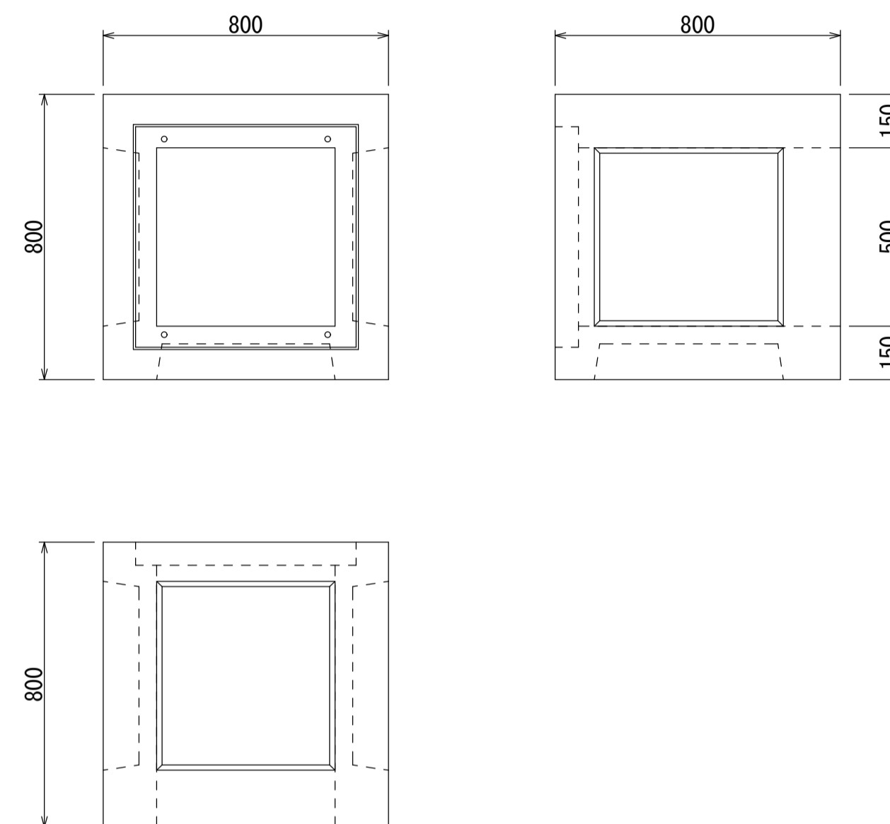
FM-500 (555kg)
