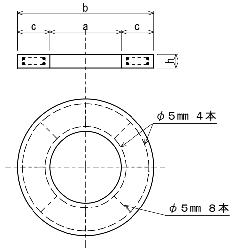
人孔調整用ブロック
