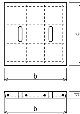
コンクリート蓋 D型
