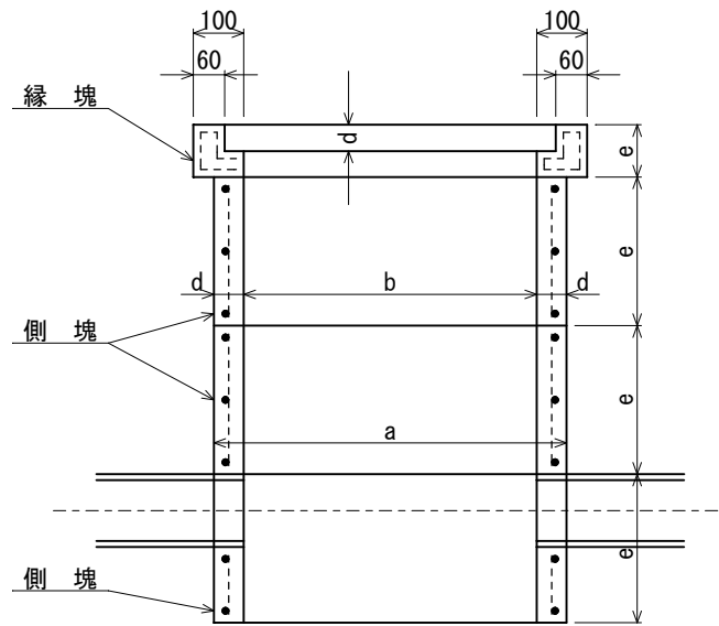
コンクリート蓋 D型
